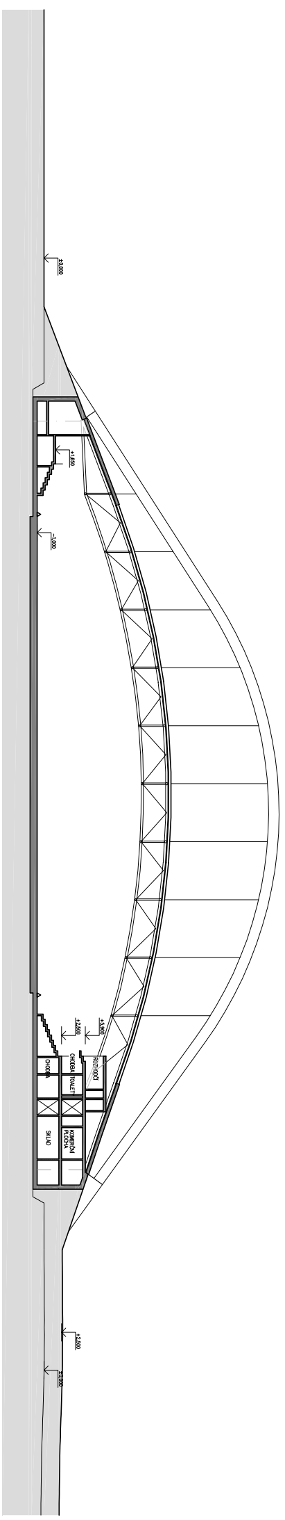
ŘEZ D
